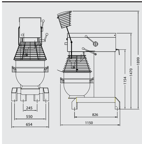
VL-1S Automatisk hastighetsreglering och kittelnedsänkning
