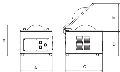
SLAM 270 - 310 - 350 SLAM 410 - 460 - 520
